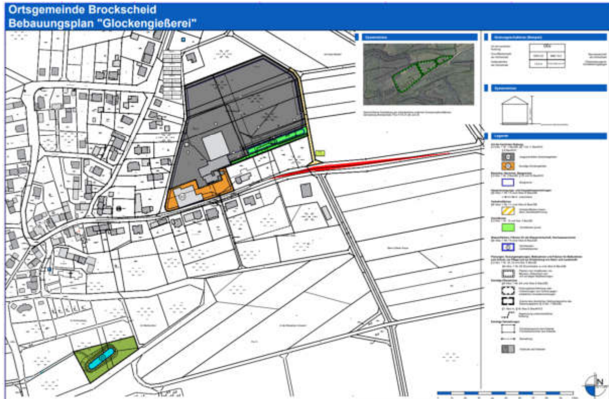
Abbildung 13: Planzeichnung
